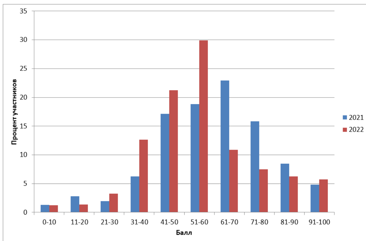
Рис. 2. Диаграмма распределения тестовых баллов по литературе в 2021-2022 г.
