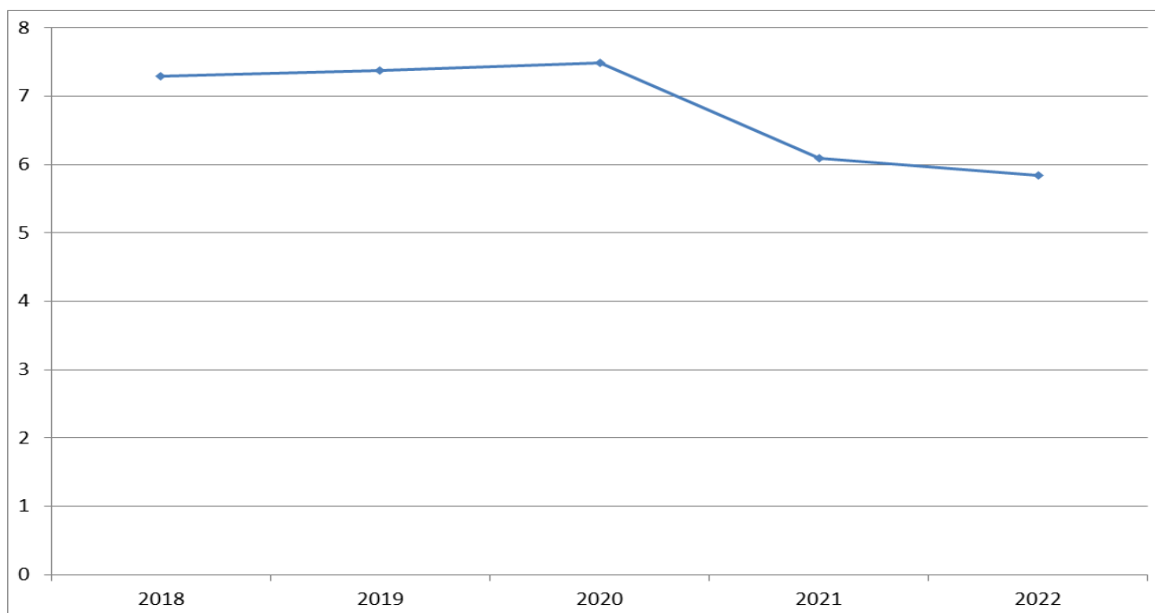
Рис. 4. Процент не преодолевших минимального порога
