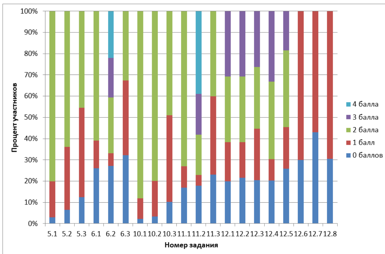
Рис. 5. Процент участников, набравших соответствующий балл за задание с развернутыми ответами (5, 6, 10, 11, 12)
