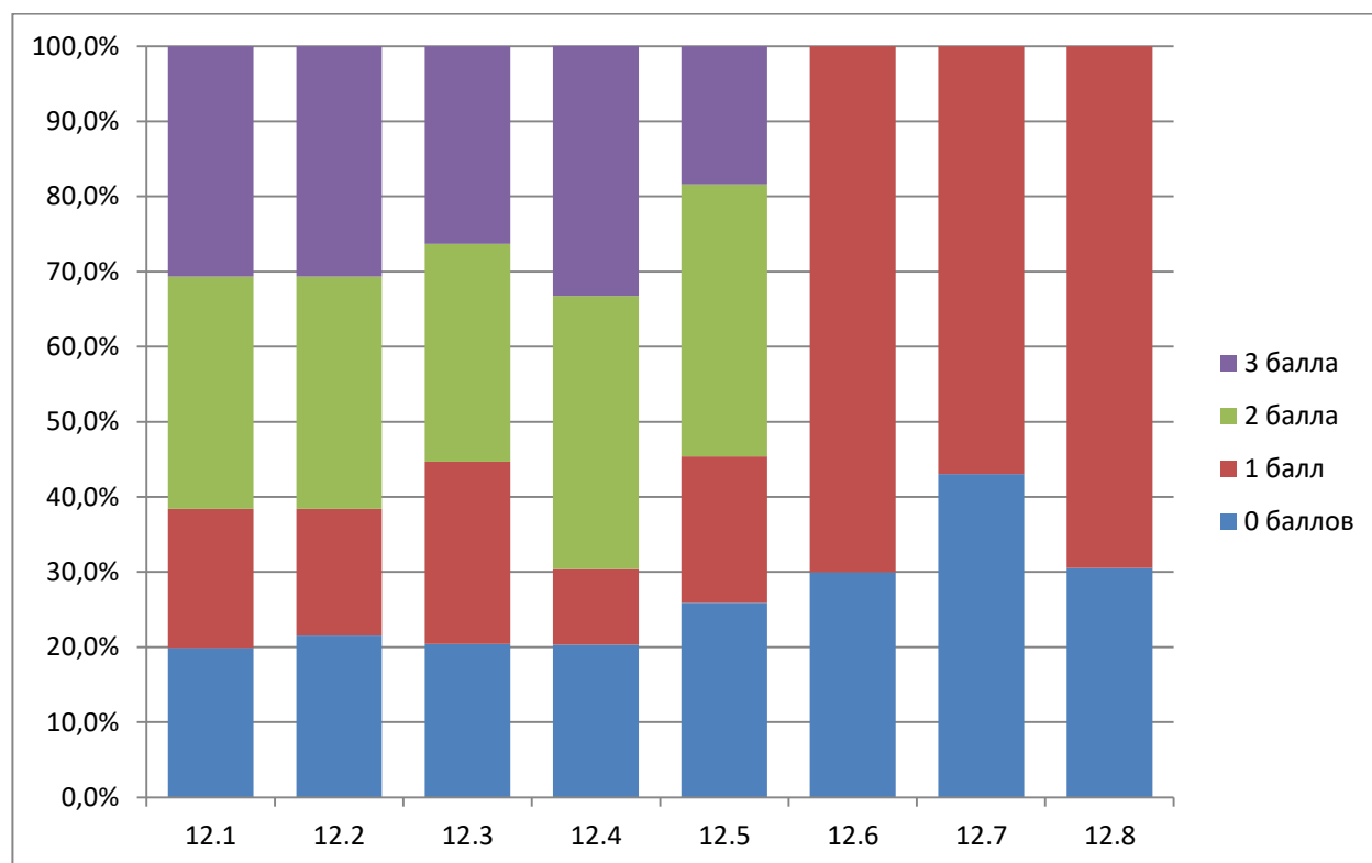
Рис. 5.1. Процент участников, набравших соответствующий балл за задание 12 с развернутыми ответами (сочинение)
