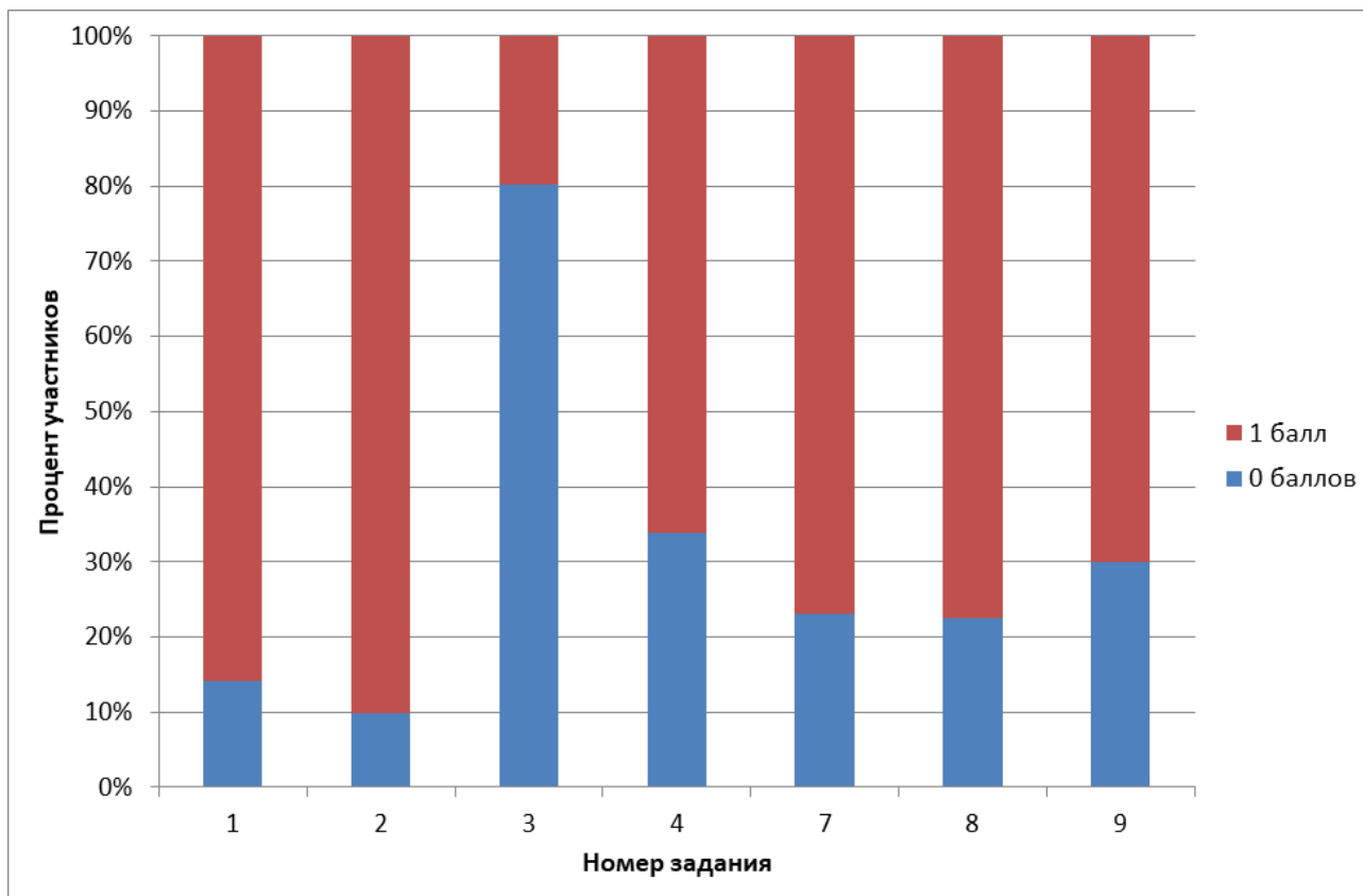
Рис. 4. Процент участников, набравших соответствующий балл за задание с краткими ответами (1-4, 7-9)
