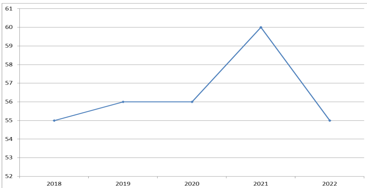
Рис. 3. Динамика среднего балла по предмету
